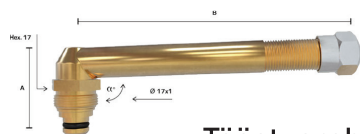
Tööstusrehvi TL-ventiil (M17x1)
